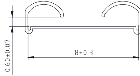
A-A KESITI
