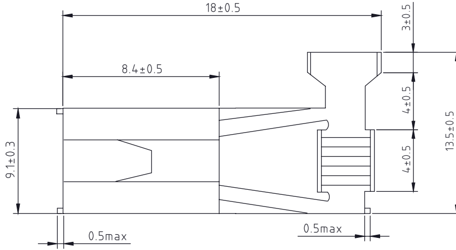
A-A KESITI
